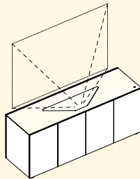
MEDIA-BACKBOARD MIT PROJEKTOR MEDIA CRENZAS WITH INTEGRATED PROJECTOR B/L: 160 / 200 / 240 H: 82 T/P: 60
